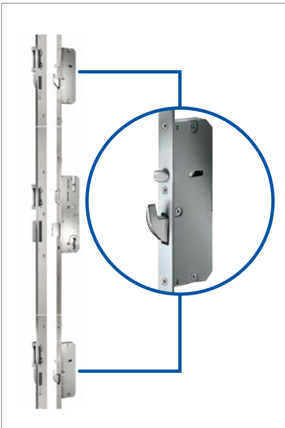
Dreifallen-Verriegelung AS 2750 Jederzeit mehr Sicherheit und dauerhafter Schutz vor Türverzug.
